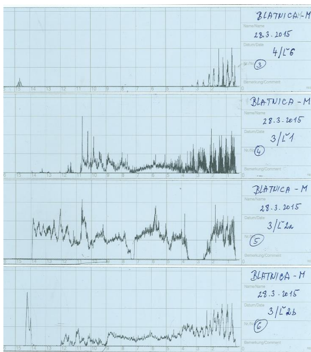
Obrázok 2 Stropy v kúrii múzea K. Plicku v Blatnici – Vrtý Resistographom z boku trámov pri záhlaviach
