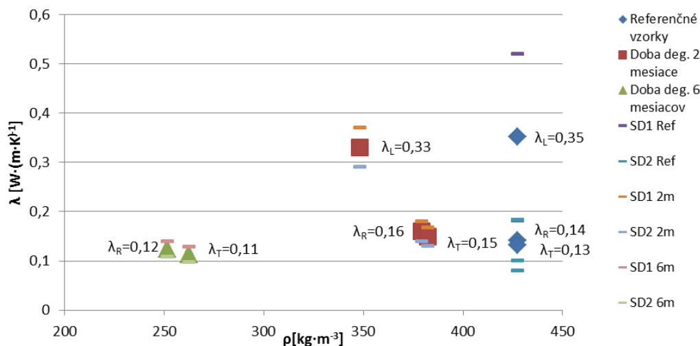
Obrázok 2 Koeficient tepelnej vodivosti dreva pre jednotlivé anatomické smery v závislosti od hustoty dreva v klimatizovanom stave ( t = 20 \pm 4 \text{ °C} ; \phi = 65 \pm 5 \% )
